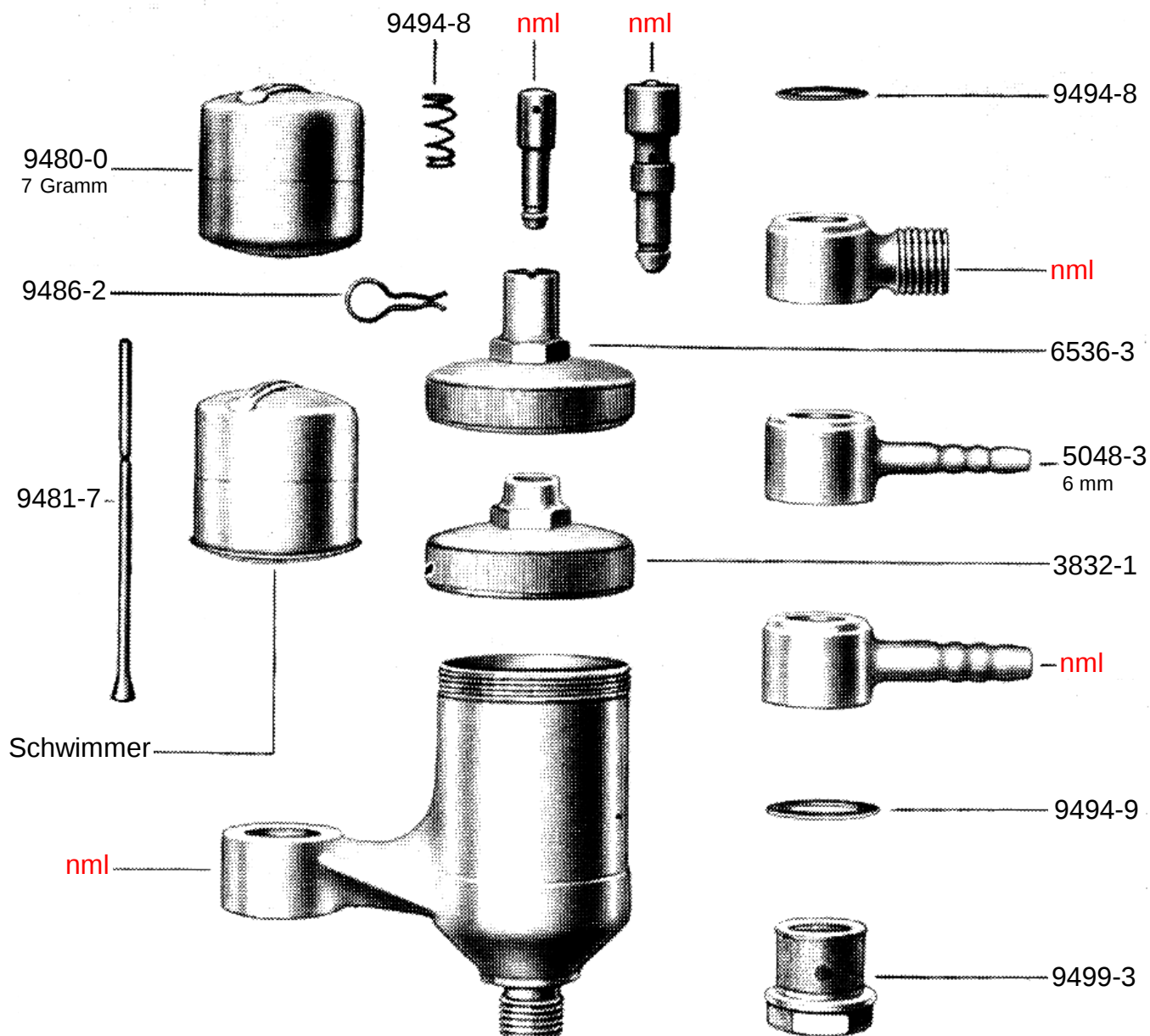
Bing Vergaserteile für Hercules OHV 500
